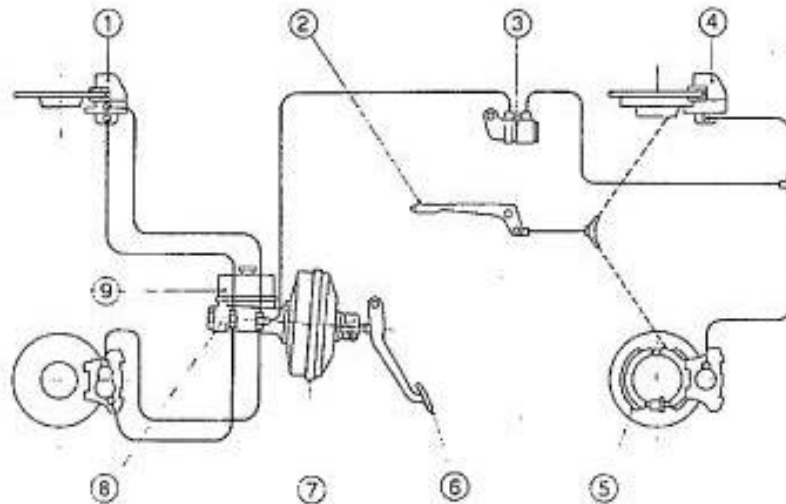
Fig. 25. - Système de freinage superduplex.
