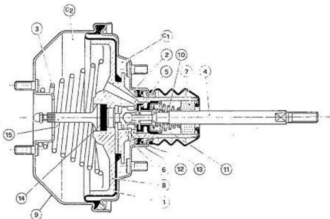
Fig. 26. - Coupe du servo-frein.
