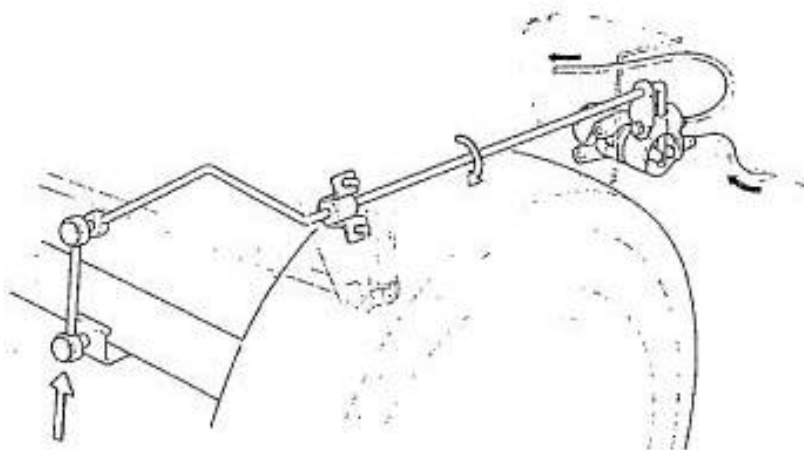
Fig. 28. - Mécanisme de commande du régulateur de freinage.
