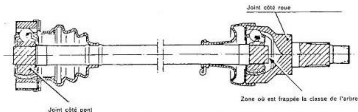
Fig. 20. - Arbre de roue avec ses joints.
