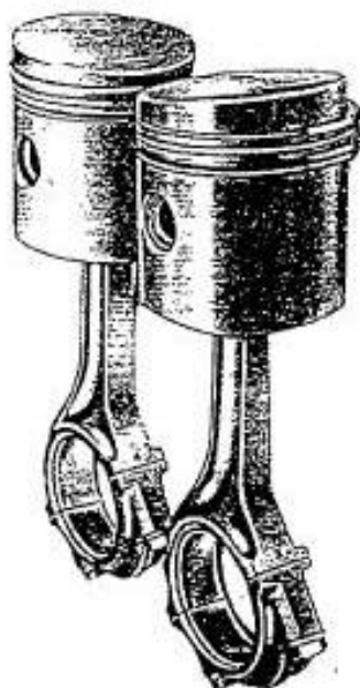
Fig. 5. - Montage correct des pistons sur les bielles.
