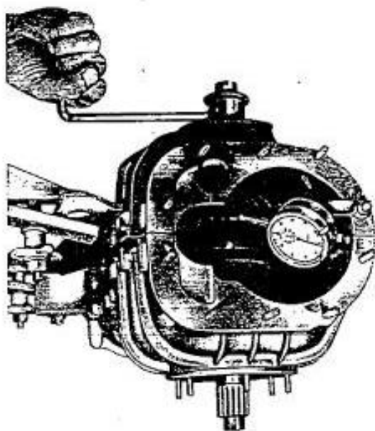
Fig. 18. - Contrôle jeu d'entre-dents pignon-couronne.
