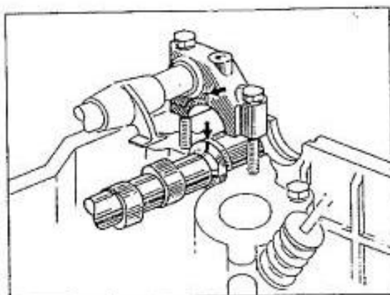
Fig. 11. - Position de montage arbres à cames.
