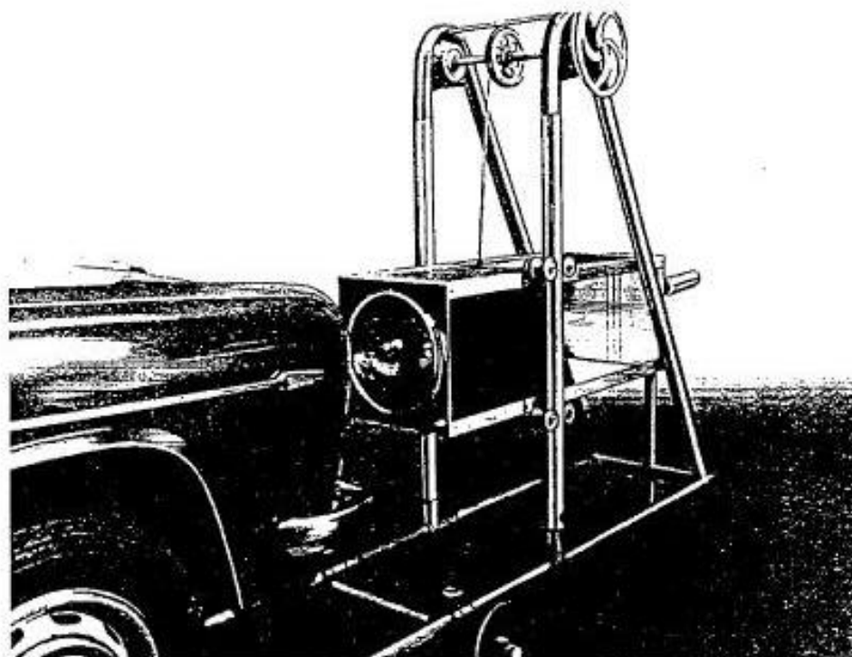
Fig. 33. - Contrôle des phares.
