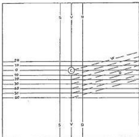
Fig. 34. - Lignes de repère pour le contrôle des phares.
