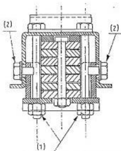
Fig. 24. - Coupe transversale du ressort à lames avant.
