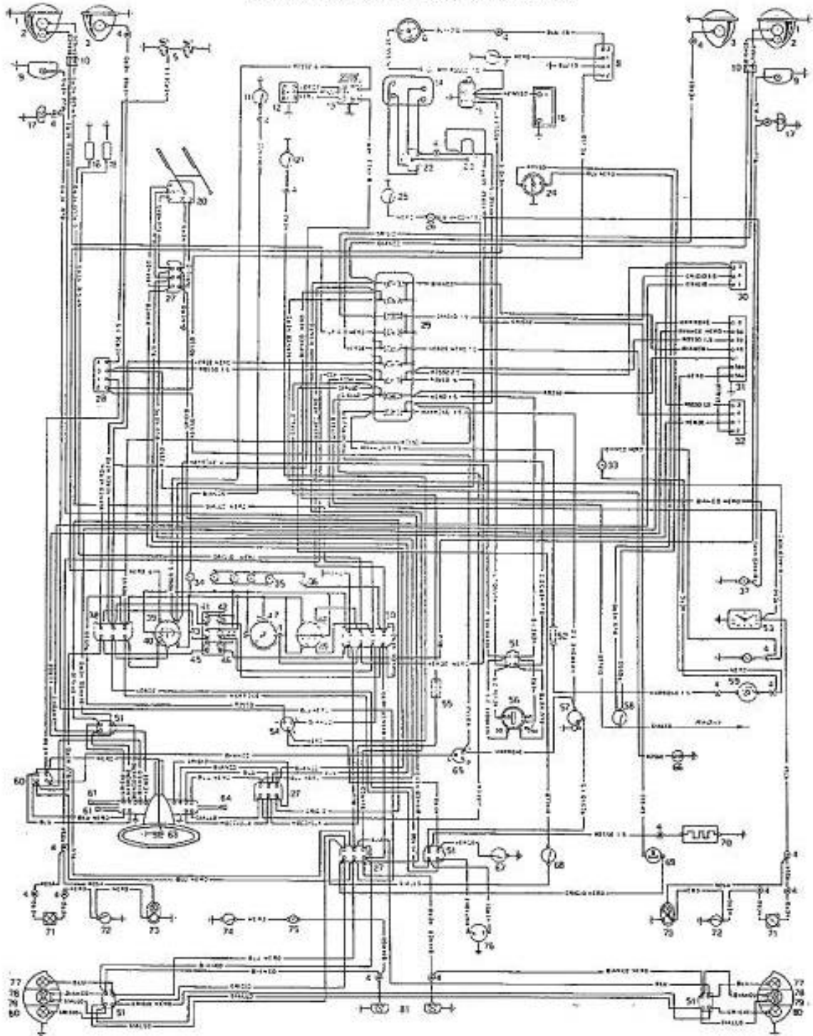
Schéma installation électrique berline (818.612).
