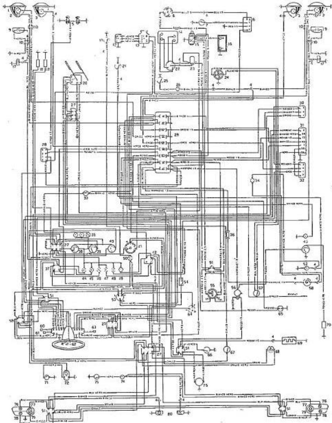
Schéma installation électrique Coupé 1600 HF (818.740).
