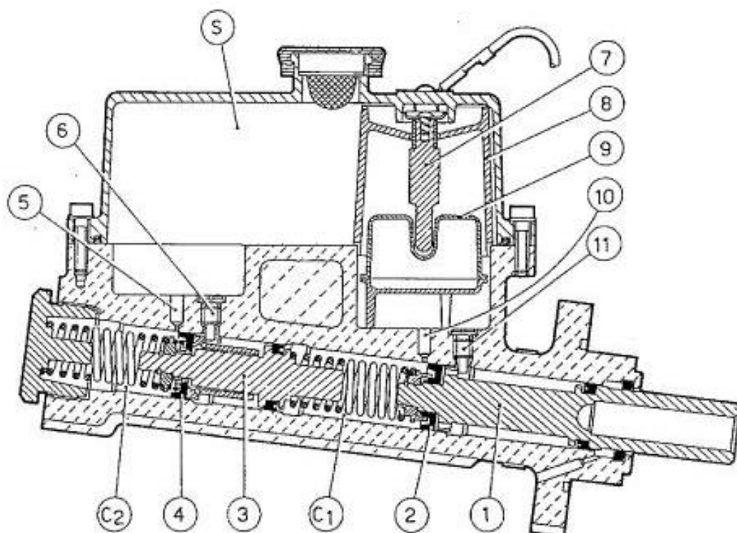
Fig. 27. - Maître-cylindre freins.
