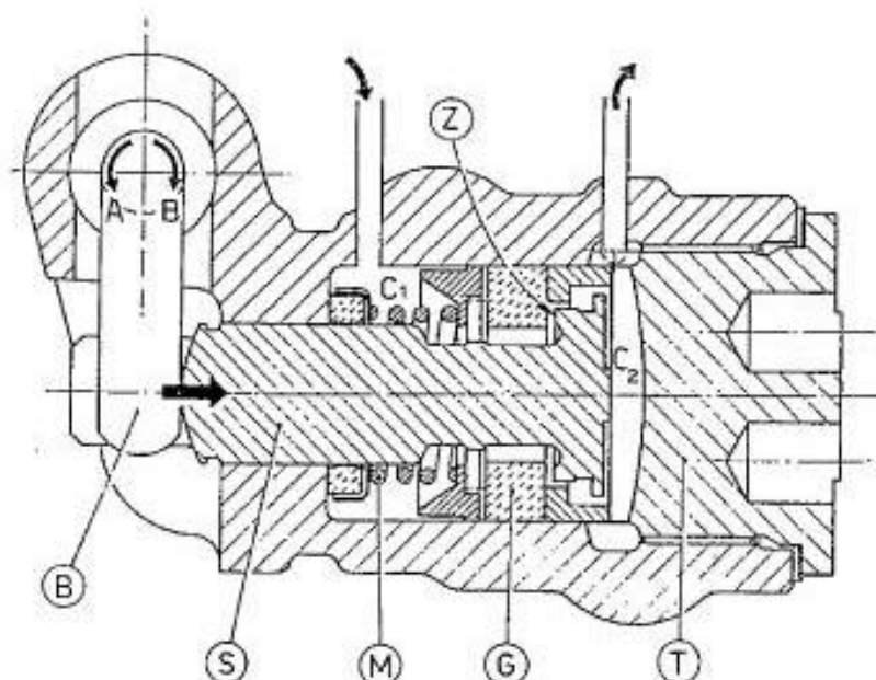
Fig. 29. - Régulateur de freinage.
