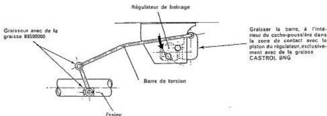
Fig. 30. - Mécanisme de commande du régulateur de freinage.
