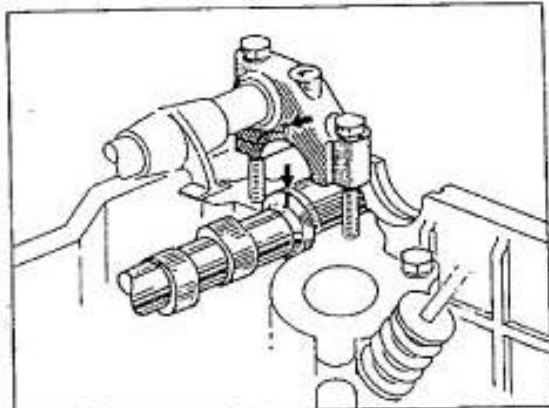
Fig. 6. - Position de montage des arbres à cames.
