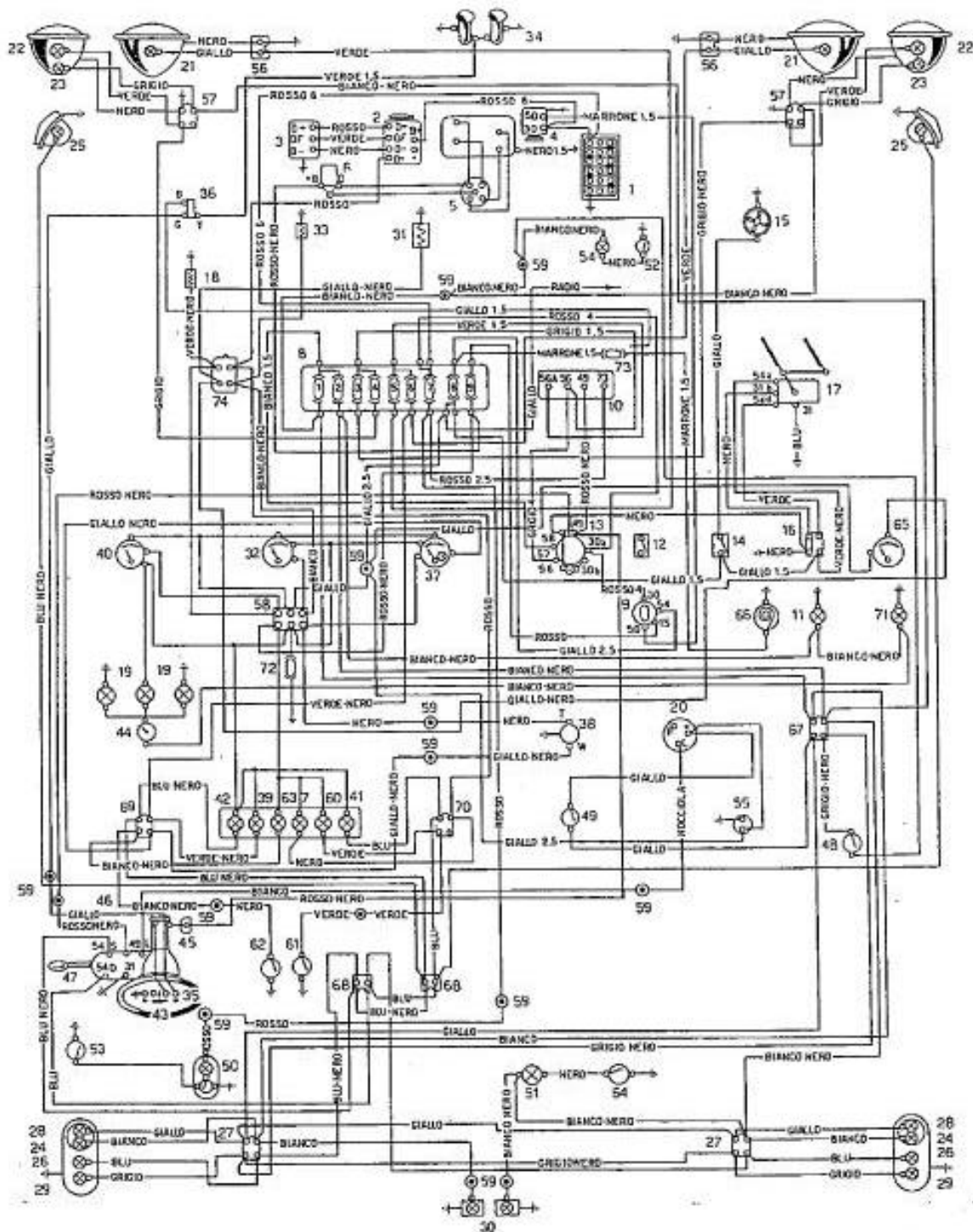
Schéma installation électrique coupé rallye 1,6 HF (818.540).
