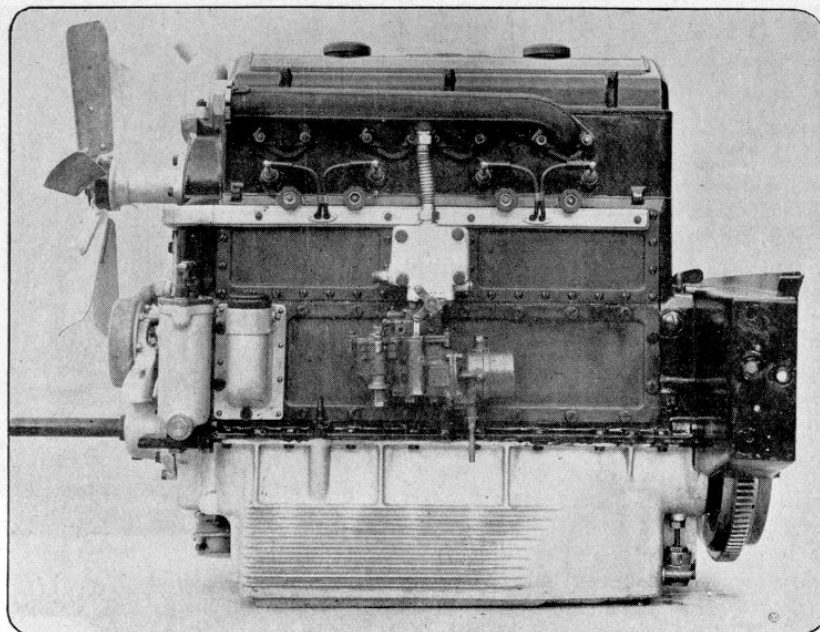
Fig. 2. — Moteur Dilambda.
